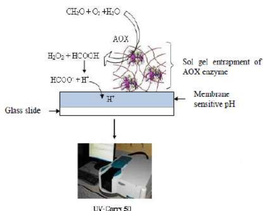
Figure 8. Formalin biosensor design (Kusuma, L. 2014)
