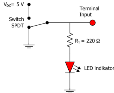
Gambar 3.6. Rangkaian Input modul dengan LED indikator
