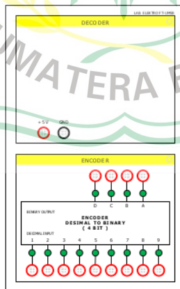
Gambar 3.10. Layot Encoder modul
