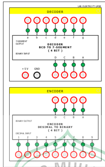
Gambar 3.12. Layout Encoder Decoder modul
