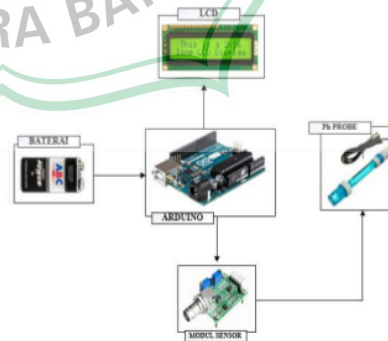
Gambar 6 Diagram Blok Sistem
