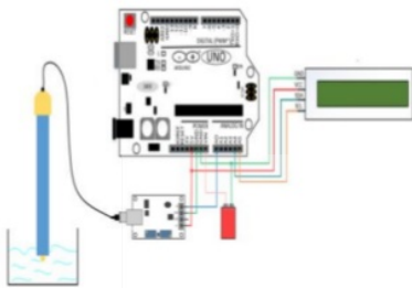
Gambar 7 Wiring Diagram Perancangan
