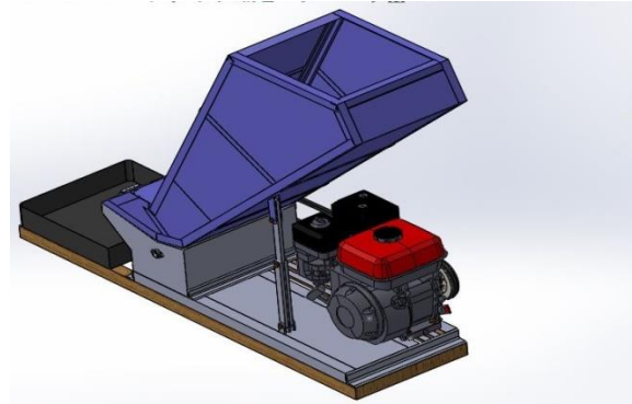
Gambar 4. 3D Modelling mesin pencacah multifungsi
