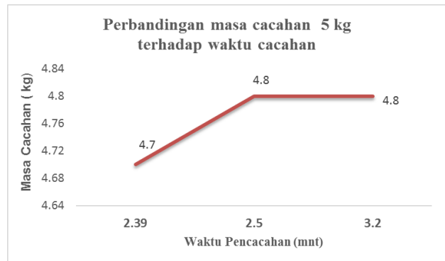
Gambar 8. Grafik perbandingan masa cacahan 5 kg terhadap waktu cacahan
